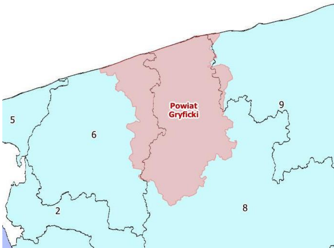
Rysunek 14. Jednolite Części Wód Podziemnych na tle Powiatu Gryfickiego
