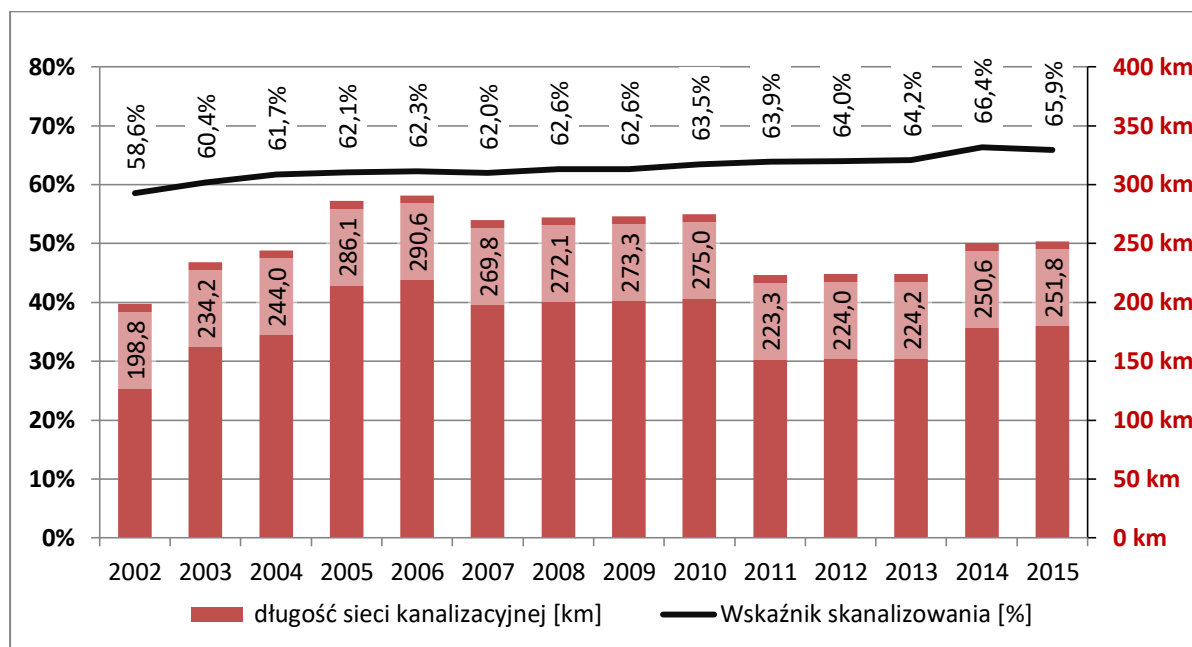
Wykres 3. Długość sieci kanalizacyjnej oraz wskaźnik skanalizowania Powiatu Gryfickiego w latach 2002 – 2015
